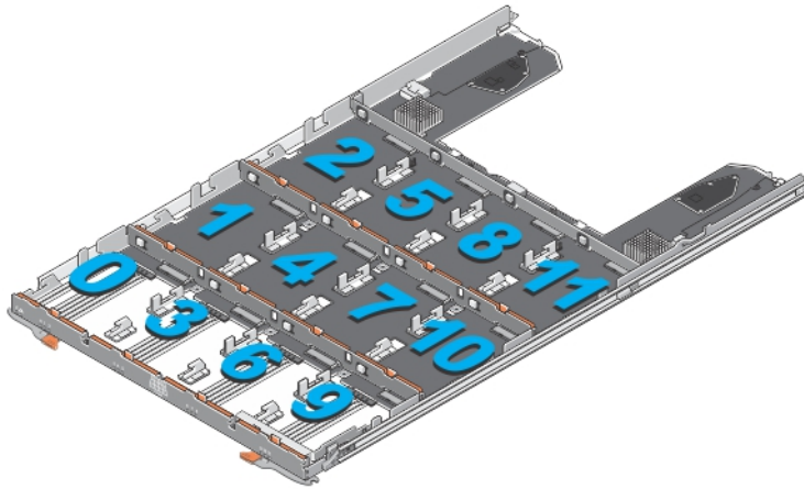
图 16: 物理磁盘盘位上的插槽编号
