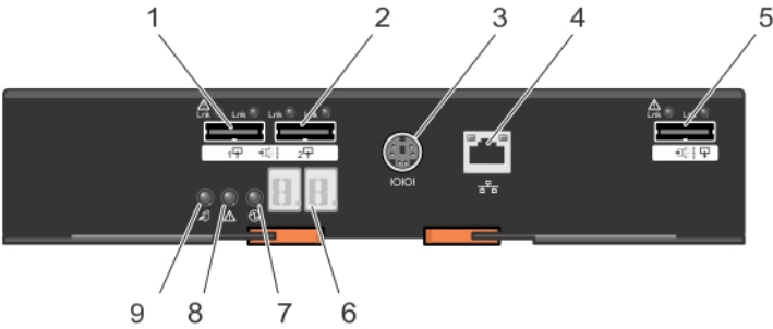
图 11: MD3060e 扩展模块部件和指示灯
