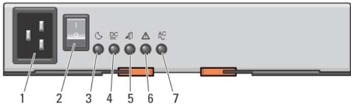
图 6: 电源设备模块部件和状态指示灯
