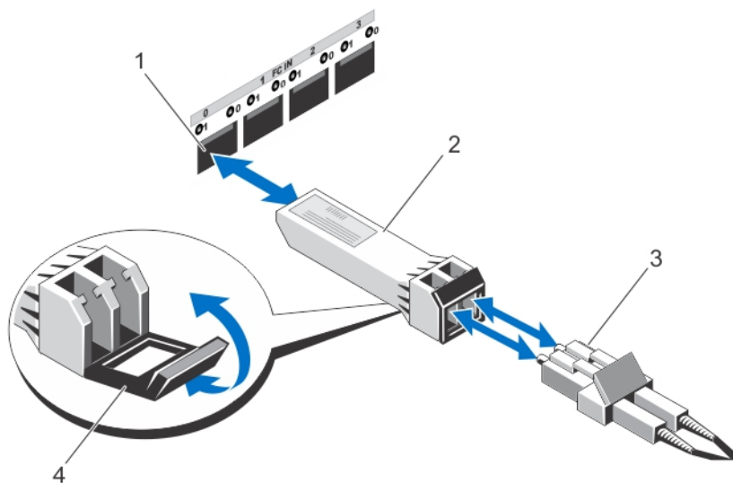
图 9: 光纤电缆连接
