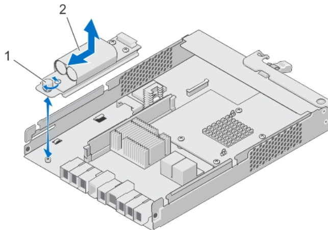
图 25: 卸下和安装 RAID 控制器模块备用电池装置
